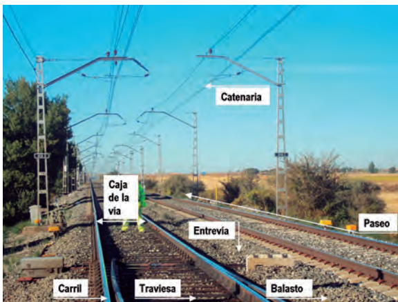
Imagen 5.1. Elementos de una vía ferroviaria. Fuente: VIAS
