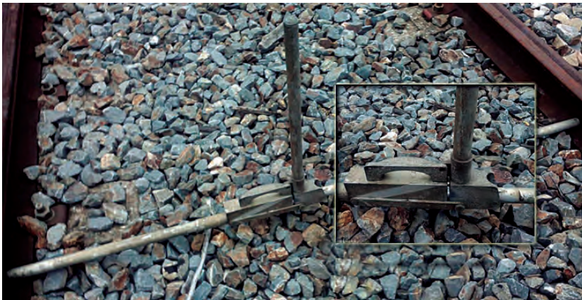
Imagen 4.3. Barra de shuntado, Fuente: Daniel Sánchez Polo
